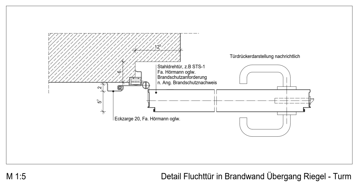
Detail Fluchttür in Brandwand Übergang Riegel - Turm
