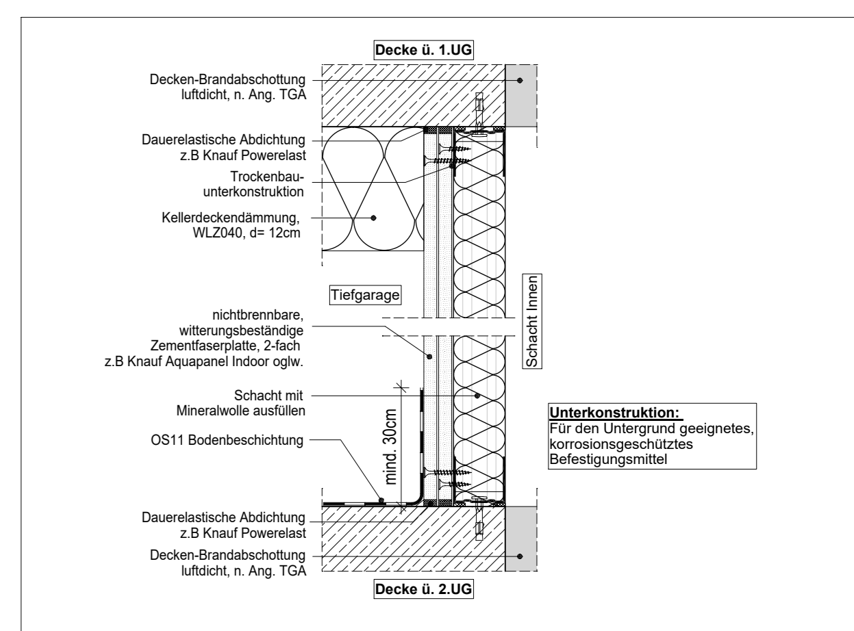
Detail Schachtverkleidung in der Tiefgarage
