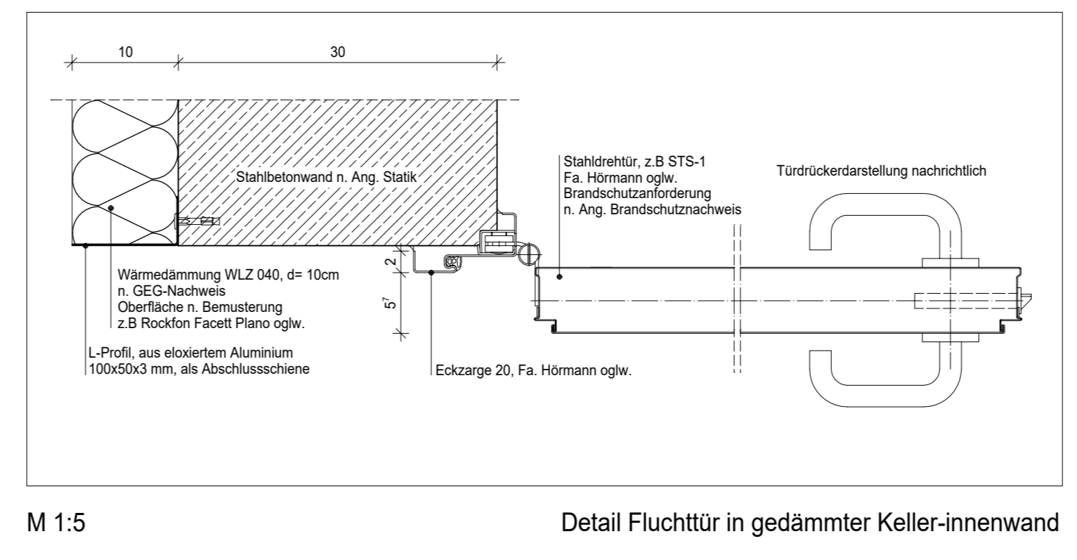
Detail Fluchttür in gedämmter Kellerinnenwand
