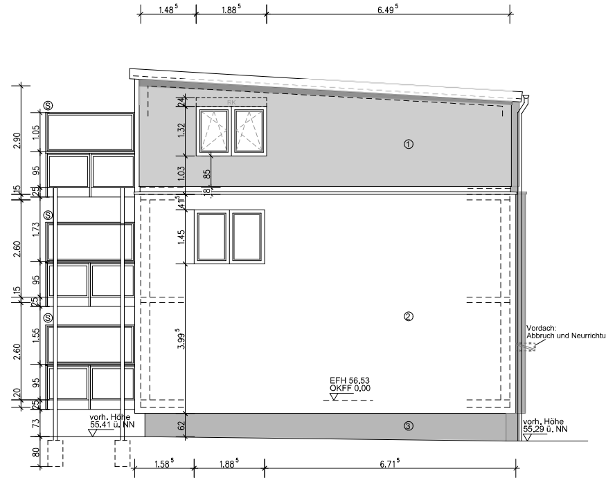
Ansicht Nord-Ost
