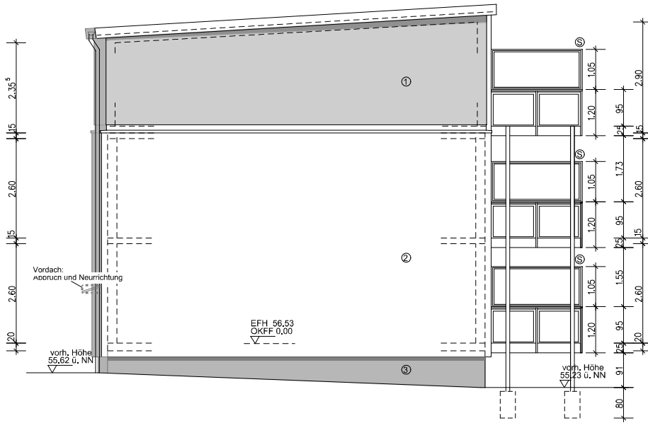
Ansicht Süd-West
